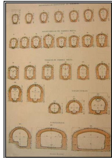
Làmina del projecte de Pere Garcia i Fària: “ Proyecto de saneamiento del subsuelo de Barcelona: alcantarillado, drenaje, residuos urbanos ” datat en 1891. En aquesta, es reproduïxen les seccions dels diferents tipus de canalitzacions emprades bàsicament a l'Eixample.
